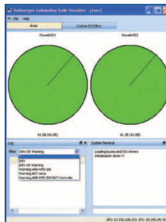
Simulator für SPS und Bewegungssteuerung
