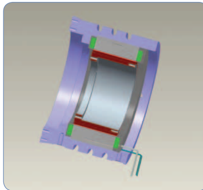
Rahmenloser rotatorischer Direktantrieb mit Wasserkühlung
