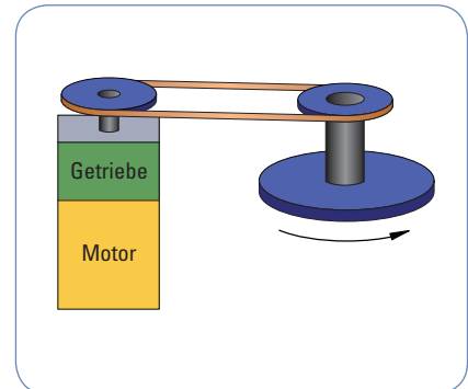
Servomotor und Getriebe
