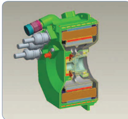
Elektrischer Anlasser/Generator, 200 kW
