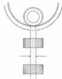
PowerTRUE™ Getriebetechnologie
