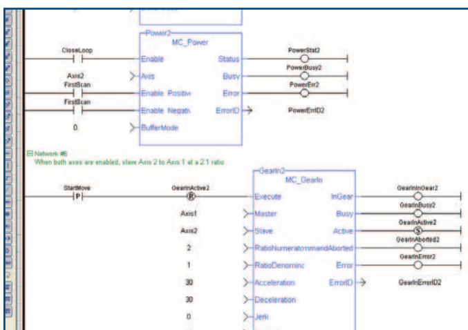
PLCopen-Beispiel
