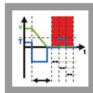
Safe Brake Control (SBC) nur mit SIL3-Karte
