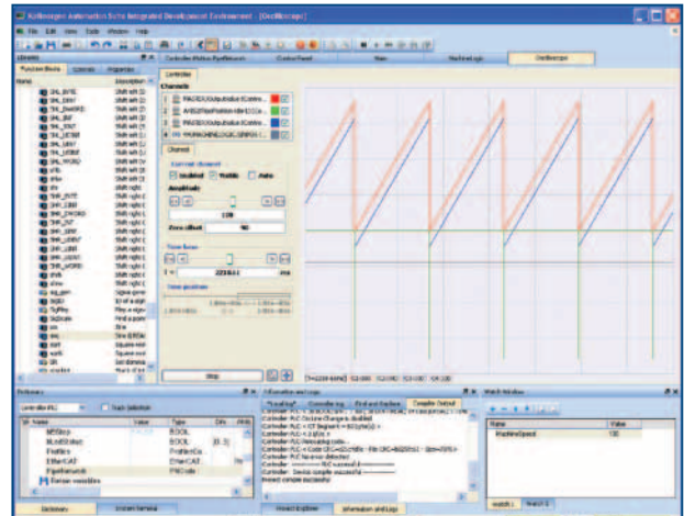
Integriertes Software-Oszilloskop
