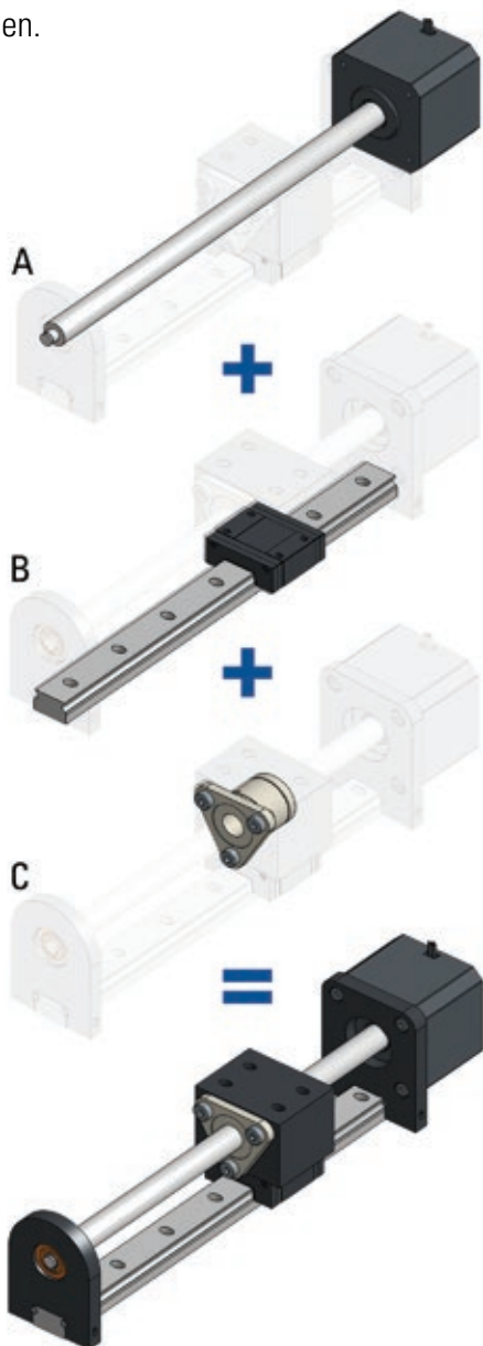
A. Thomson-Spindel und Motor (MLS) B. Thomson-Profilschiene und Schlitten C. Spielfreie Thomson-Mutter.
