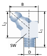
530LN45 Hydraulikschmiernippel, 45°-Winkel
