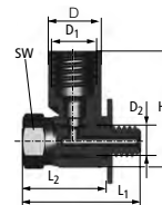
530BF... Banjo-Fittings Für Leitungen mit Außendurchmesser 530BF6 = 2,5 mm / 530BF8 = 4 mm
