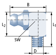
530LN90 Hydraulikschmiernippel, 90°-Winkel
