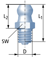
530LN Hydraulikschmiernippel, gerade 530BF6 = 2,5 mm / 530BF8 = 4 mm
